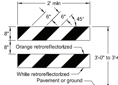
TYPE II BARRICADE
